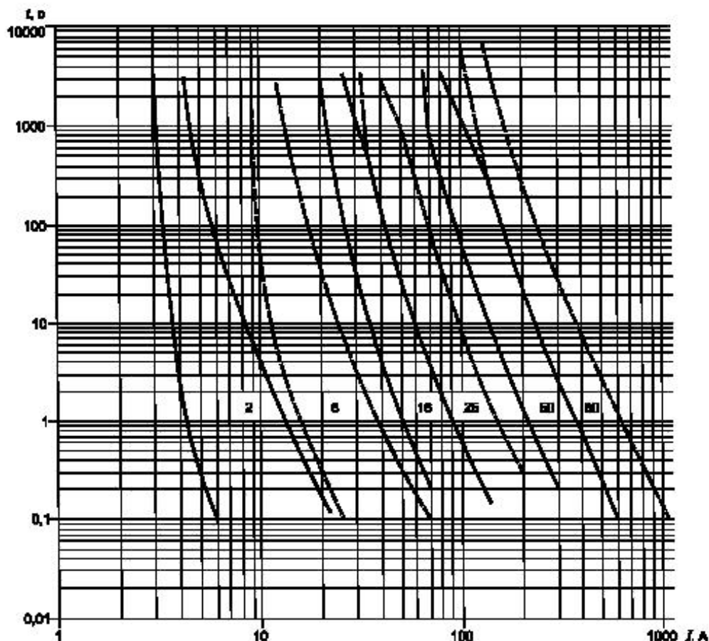
Рисунок А.1 — Время-токовые зоны для плавкого предохранителя
